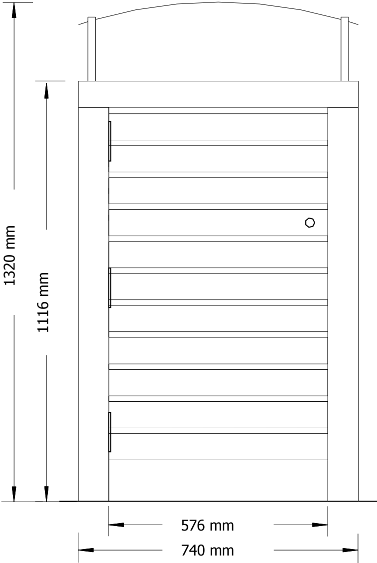
end elevation
